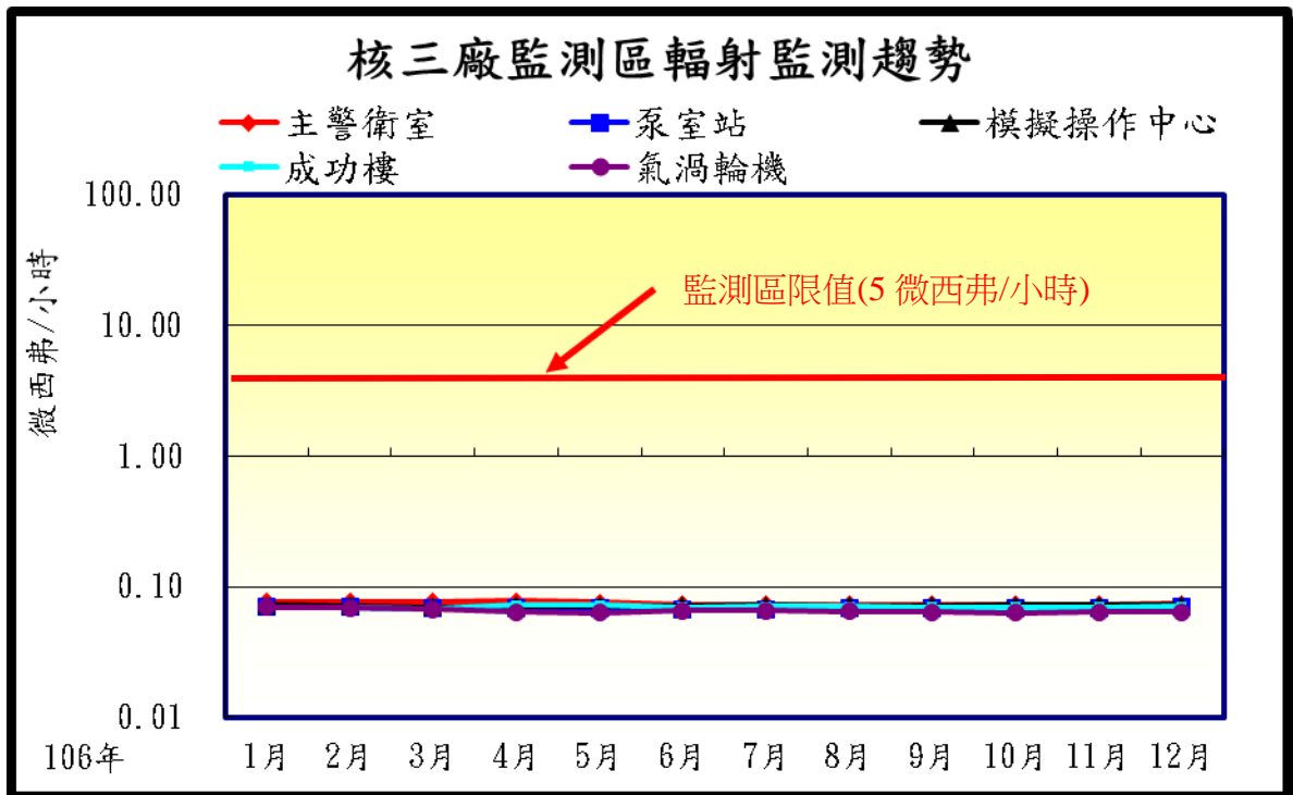
圖 4 監測區連續輻射監測趨勢
