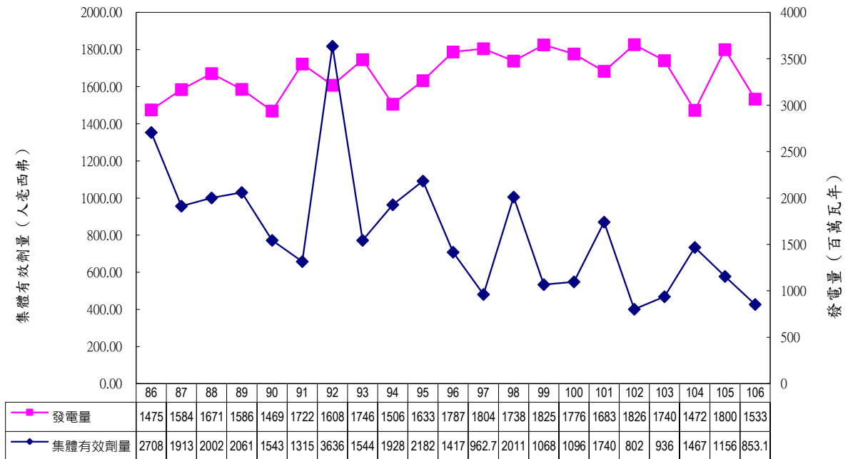
圖 8 歷年工作人員集體有效劑量與發電量比較圖
