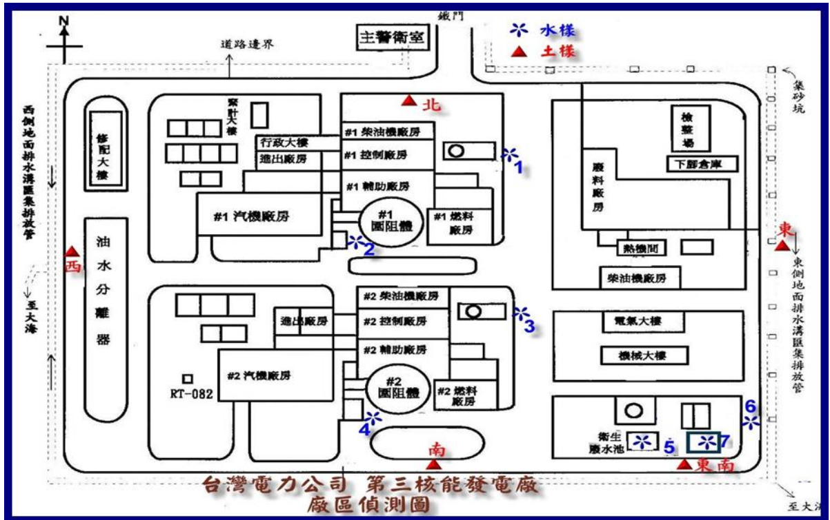
圖 6 監測區監測取樣位置 (主警衛室內)
