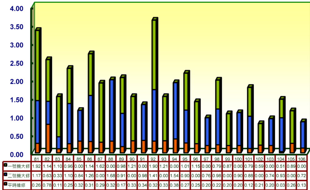
圖 7 歷年工作人員集體有效劑量統計圖
