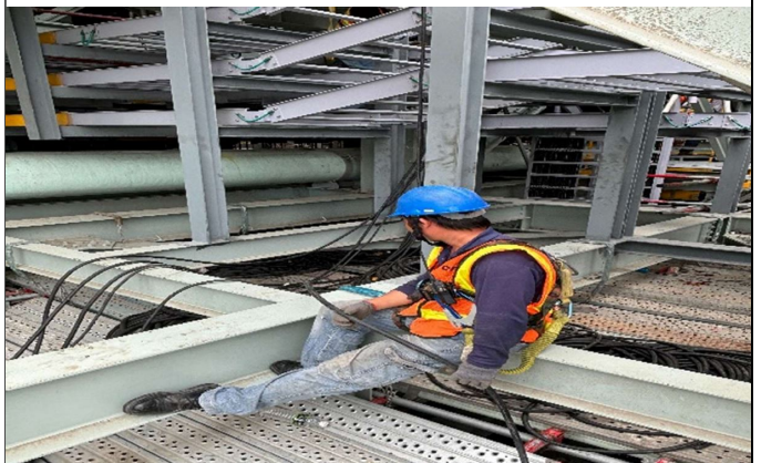
主發電設備工程 Unit 1 MPR 拉接線
