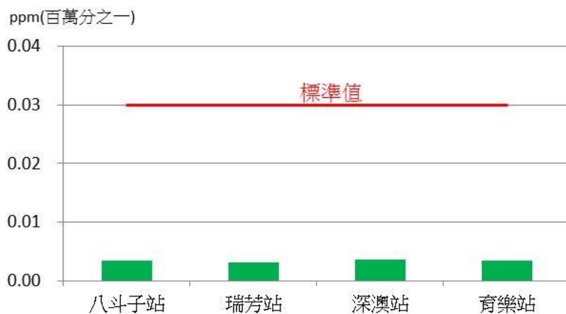
102年度二氧化硫監測結果
