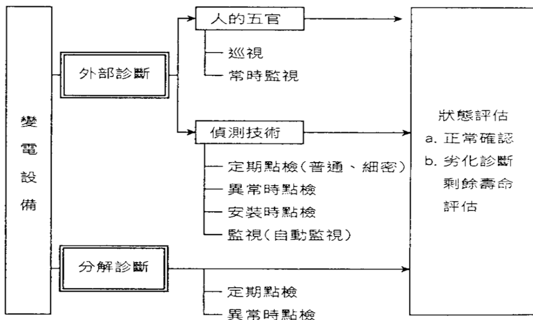
圖2-1 變電設備診斷之基本架構
