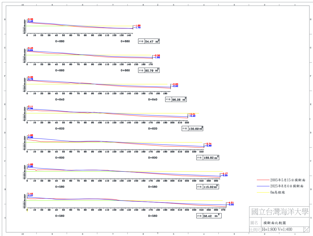
圖 4-5(b) 2025 年 8 月 4 日 B 監測區橫斷面比較圖
