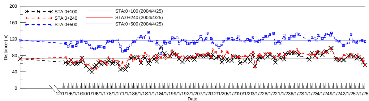
圖 4-21 岸線斷面沙灘寬度變化圖(2025/08/04)
