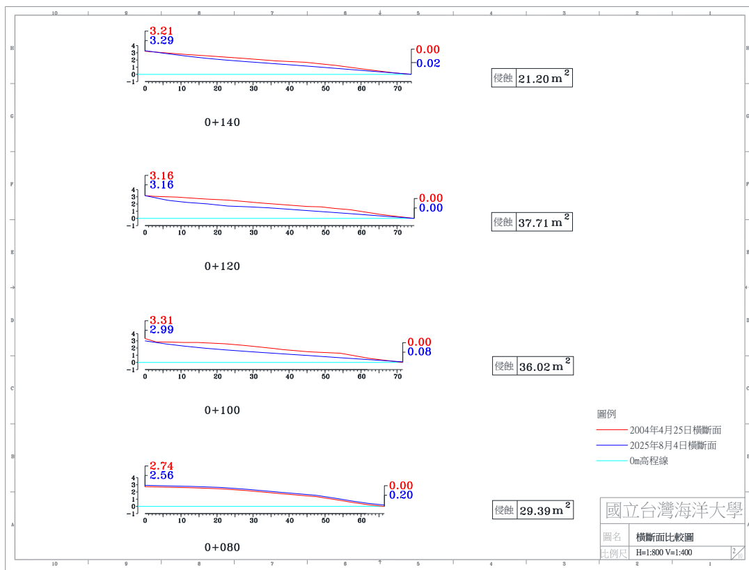
圖 4-4(i) 2025 年 8 月 4 日 A 監測區橫斷面比較圖
