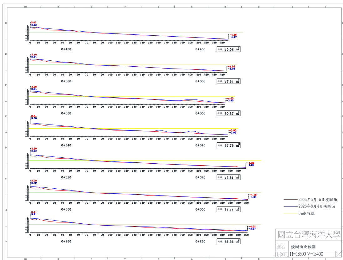
圖 4-5(d) 2025 年 8 月 4 日 B 監測區橫斷面比較圖
