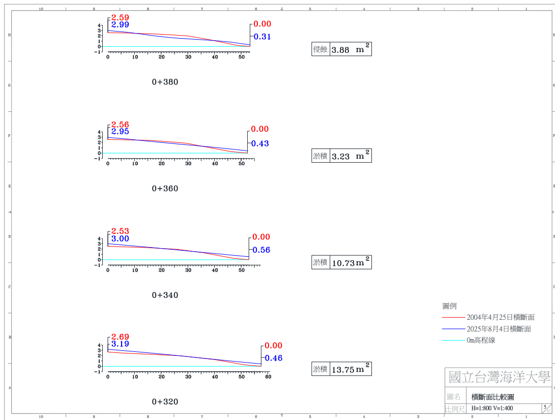
圖 4-4(f) 2025 年 8 月 4 日 A 監測區橫斷面比較圖
