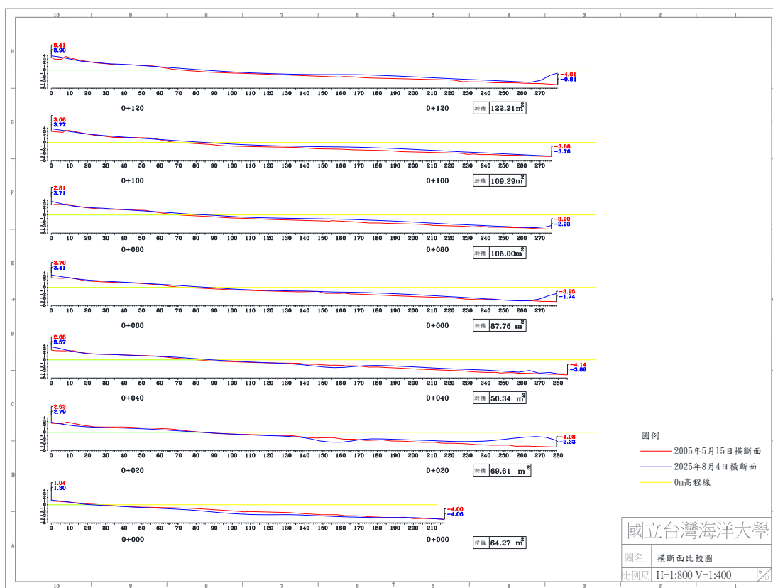
圖 4-5(f) 2025 年 8 月 4 日 B 監測區橫断面比較圖
