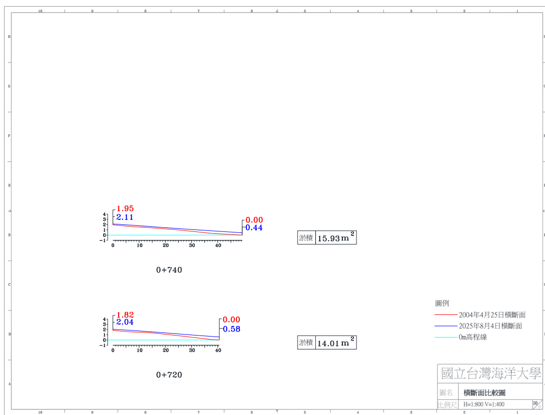
圖 4-4(a) 2025 年 8 月 4 日 A 監測區橫斷面比較圖
