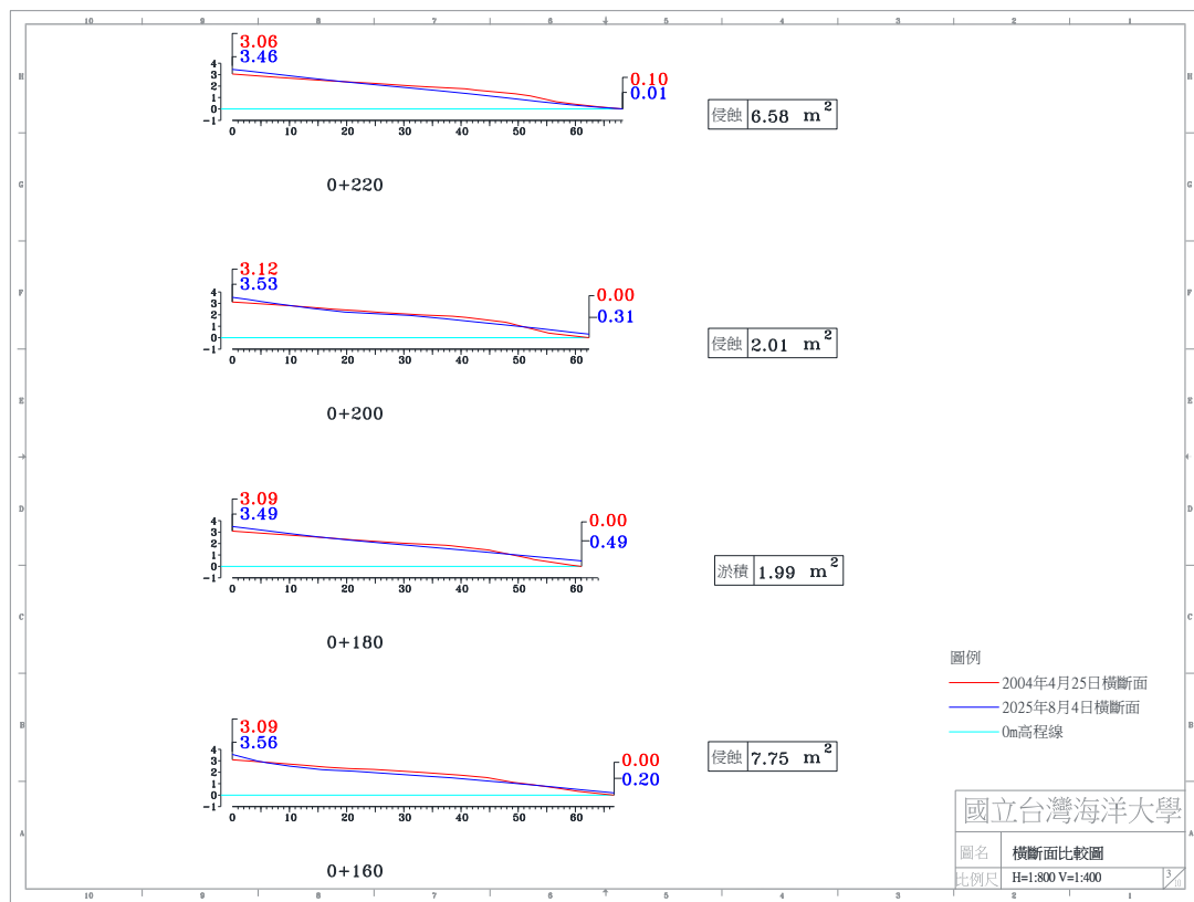
圖 4-4(h) 2025 年 8 月 4 日 A 監測區橫斷面比較圖
