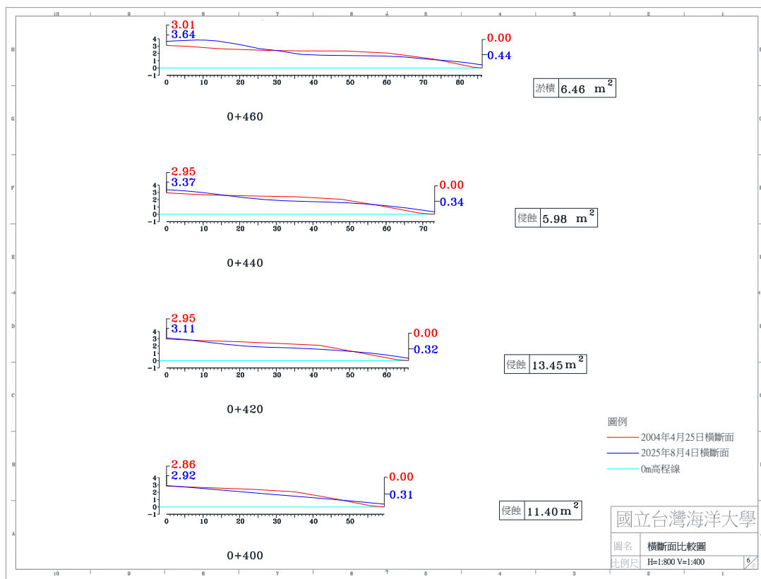
圖 4-4(e) 2025 年 8 月 4 日 A 監測區橫斷面比較圖
