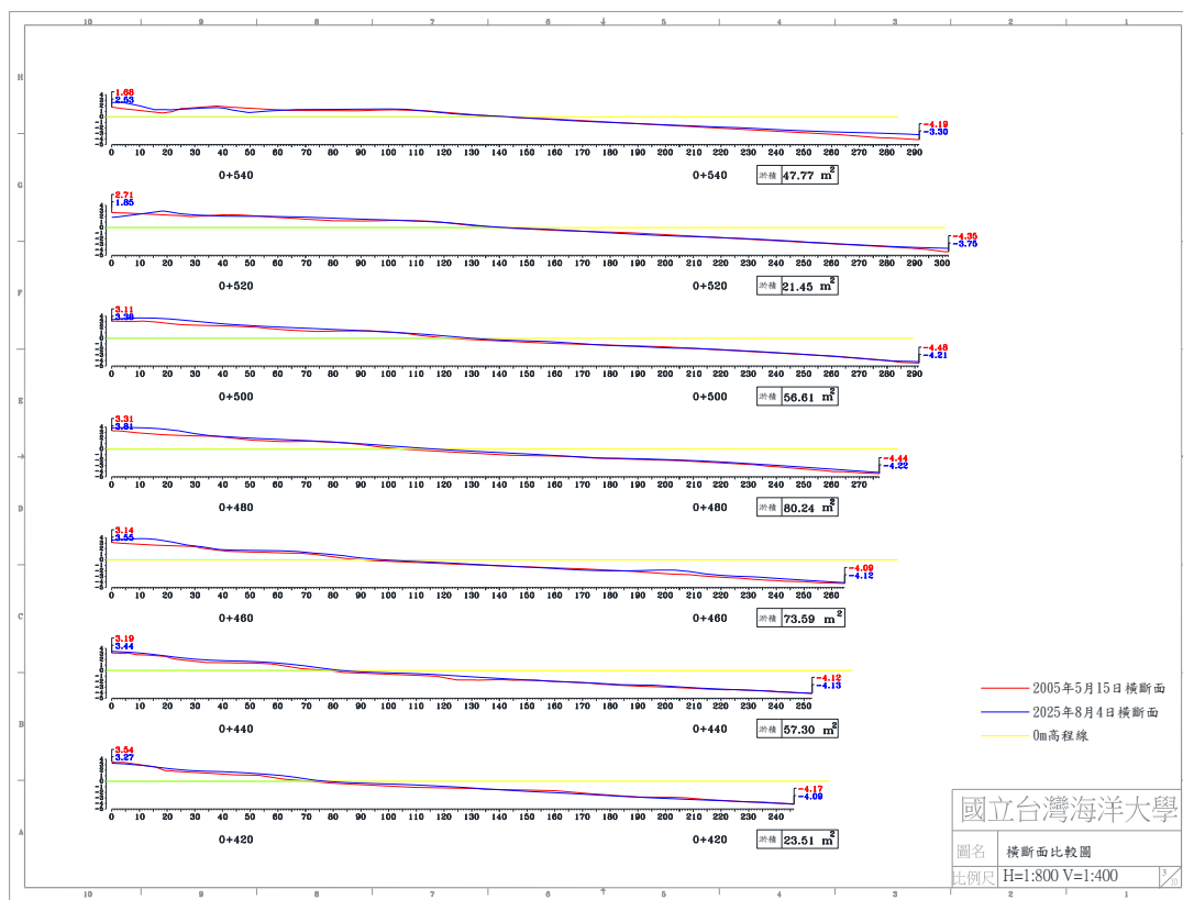
圖 4-5(c) 2025 年 8 月 4 日 B 監測區橫斷面比較圖
