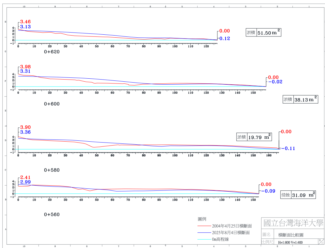
圖 4-4(c) 2025 年 8 月 4 日 A 監測區橫斷面比較圖
