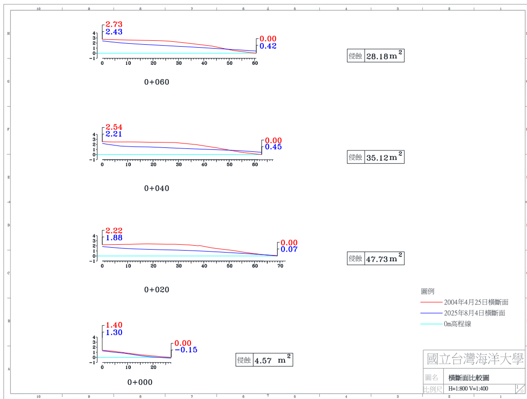
圖 4-4(j) 2025 年 8 月 4 日 A 監測區橫斷面比較圖
