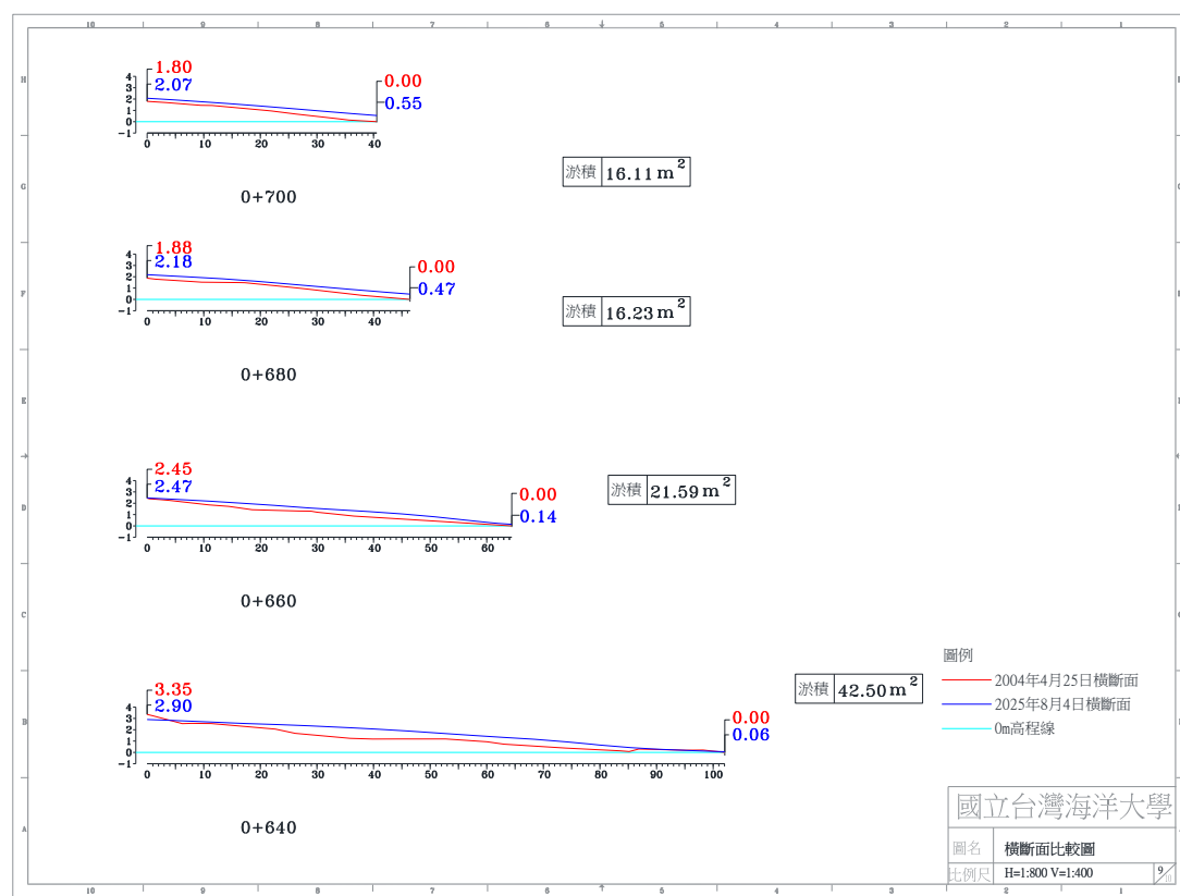
圖 4-4(b) 2025 年 8 月 4 日 A 監測區橫斷面比較圖
