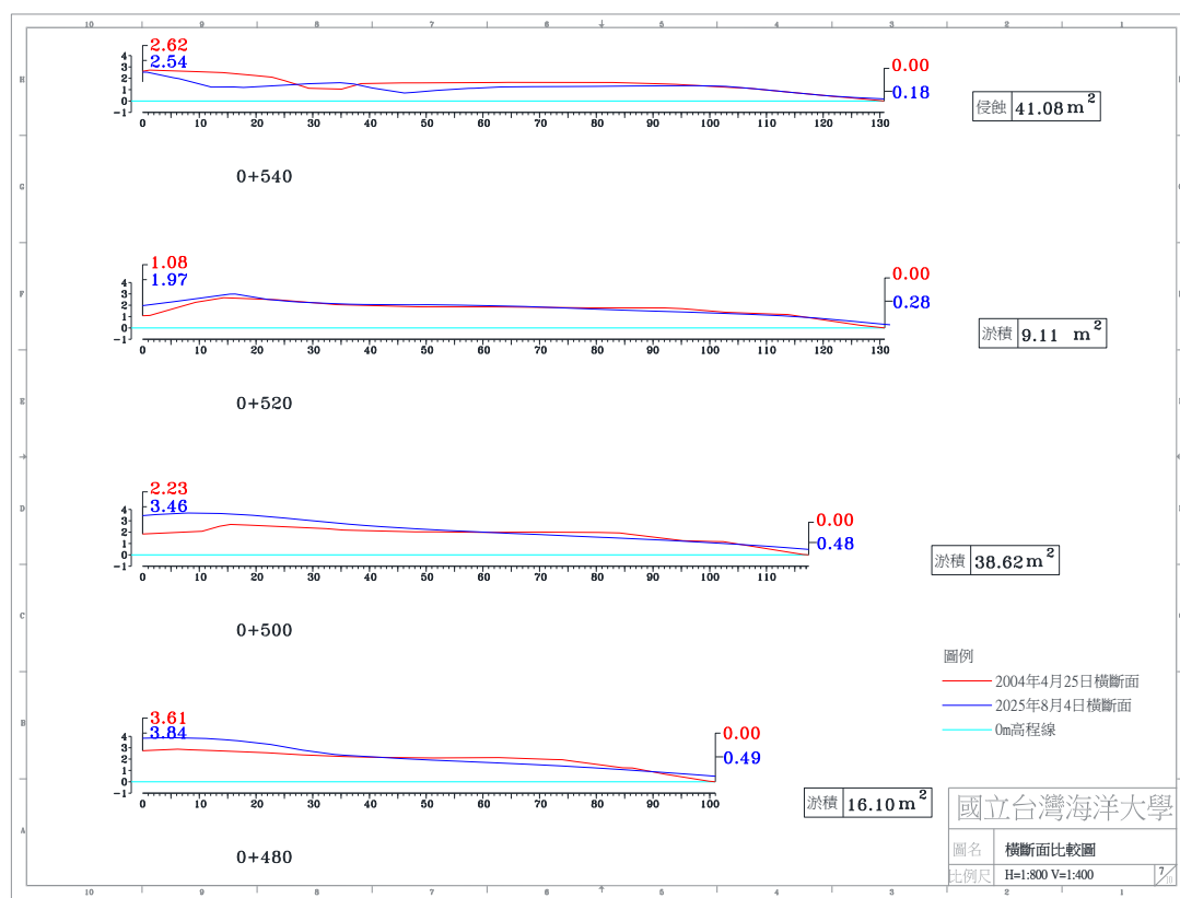
圖 4-4(d) 2025 年 8 月 4 日 A 監測區橫斷面比較圖
