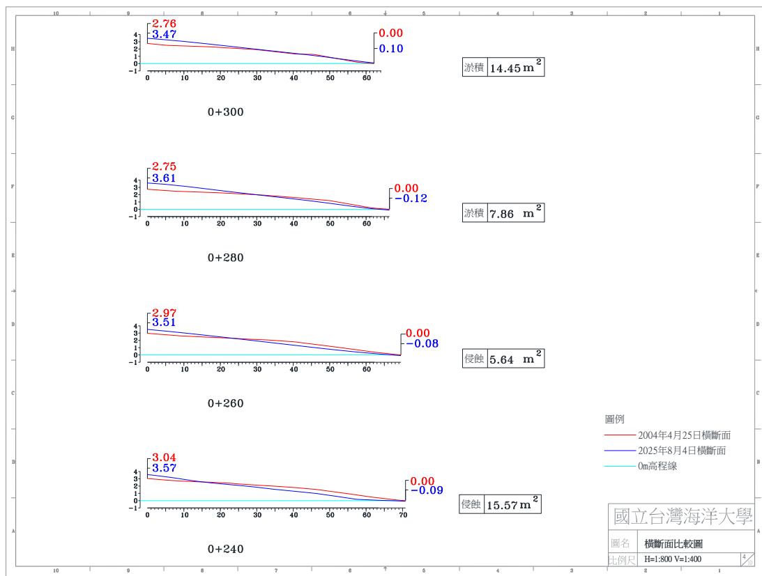
圖 4-4(g) 2025 年 8 月 4 日 A 監測區橫斷面比較圖
