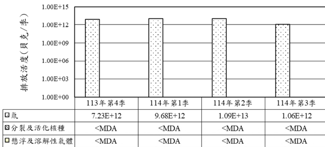
圖八 核三廠放射性廢水排放統計圖 (兩部機)
