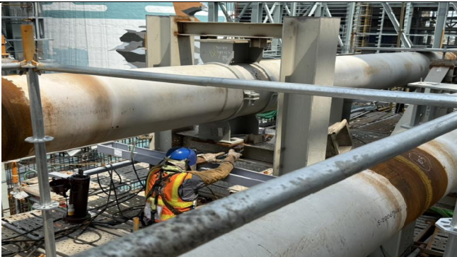
主發電設備工程 Unit 3 HRSG 副樓配管
