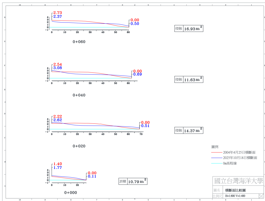
圖 4-4(j) 2025 年 10 月 18 日 A 監測區橫斷面比較圖
