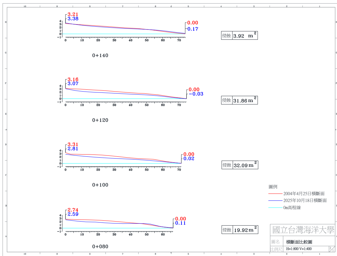
圖 4-4(i) 2025 年 10 月 18 日 A 監測區橫斷面比較圖
