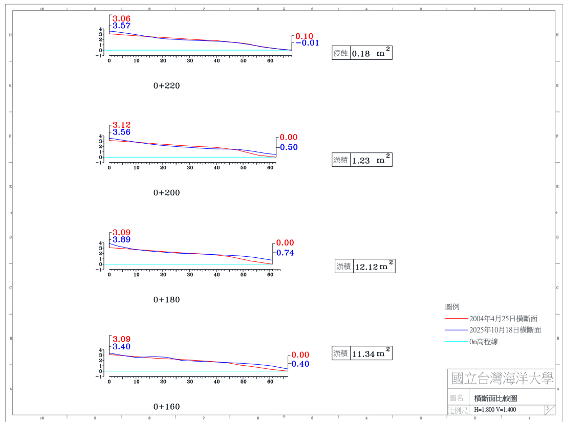
圖 4-4(h) 2025 年 10 月 18 日 A 監測區橫斷面比較圖
