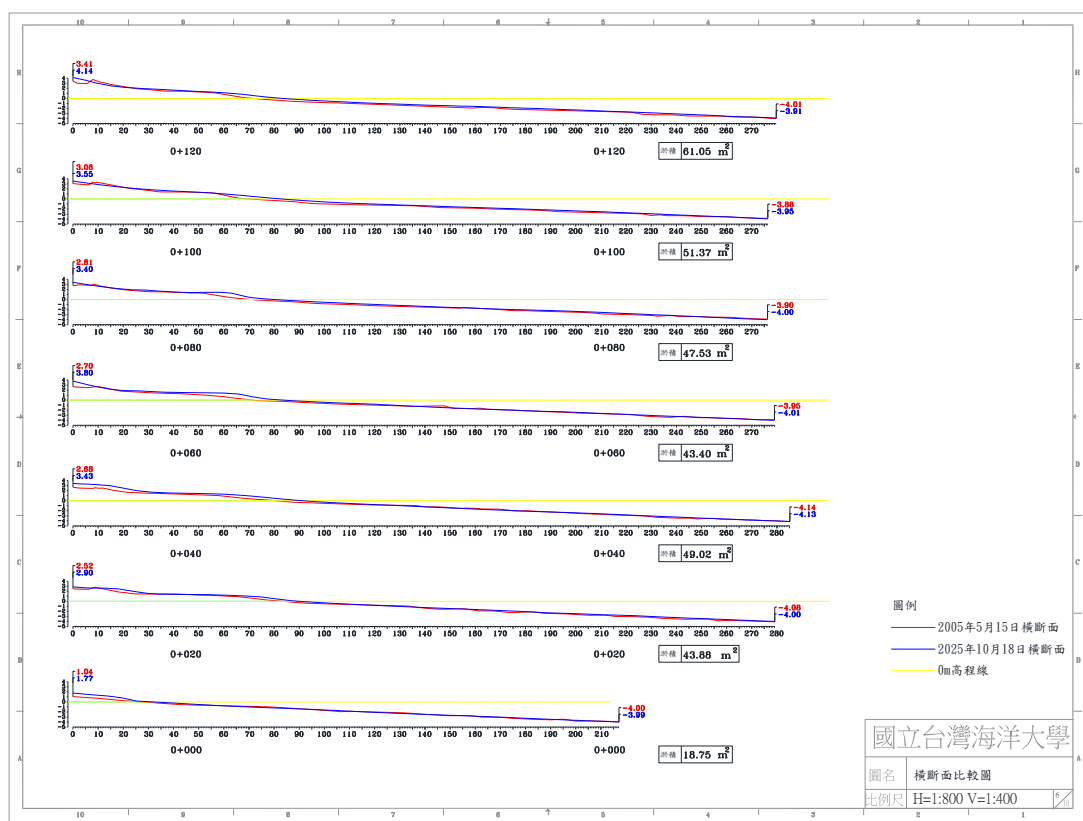
圖 4-5(f) 2025 年 10 月 18 日 B 監測區橫斷面比較圖
