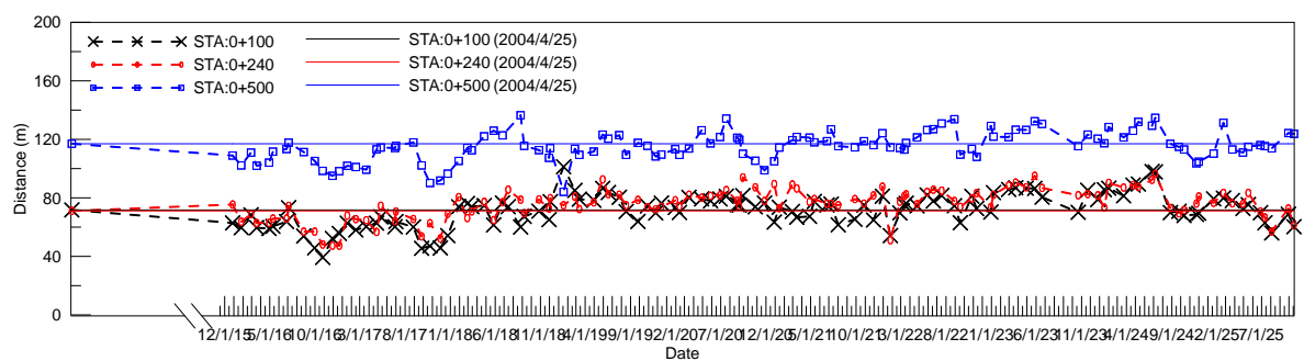
圖 4-21 岸線斷面沙灘寬度變化圖(2025/10/18)
