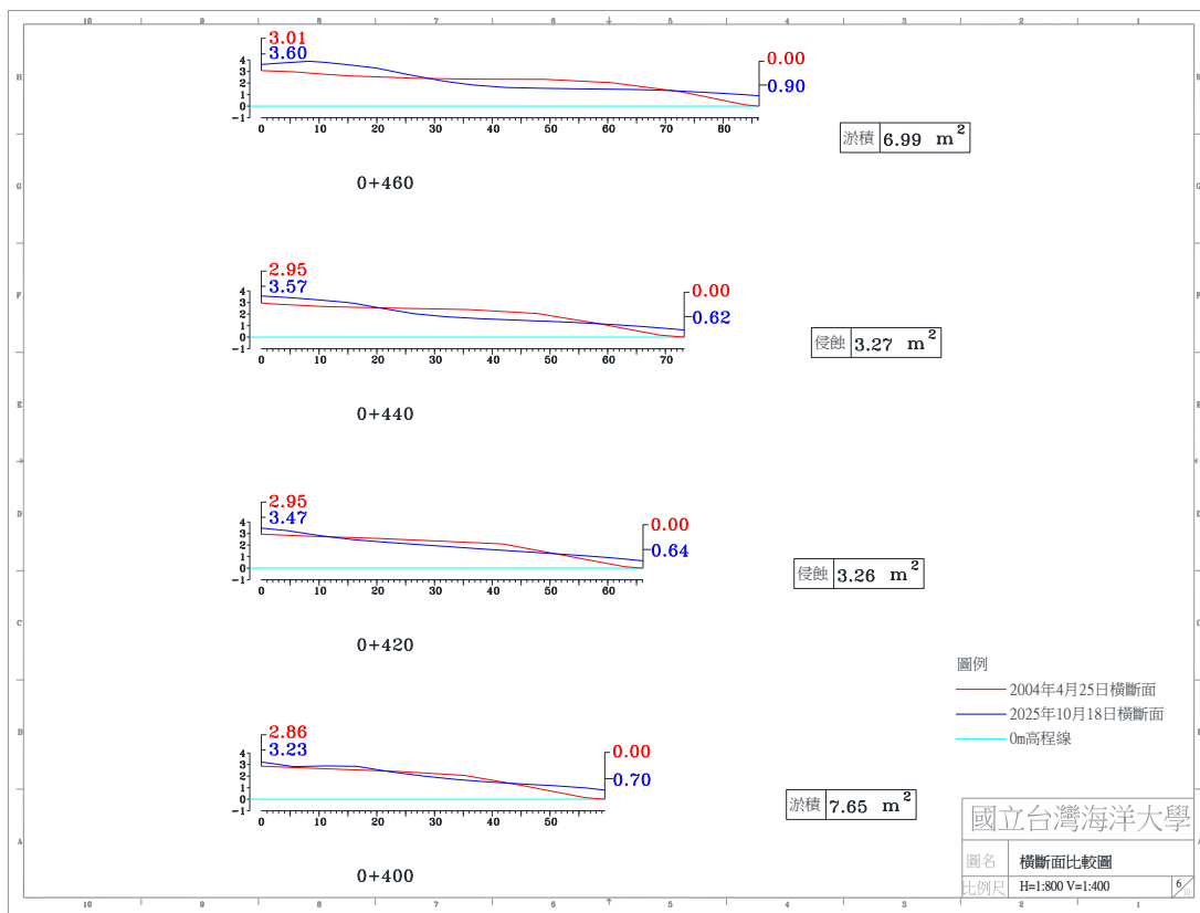
圖 4-4(e) 2025 年 10 月 18 日 A 監測區橫斷面比較圖
