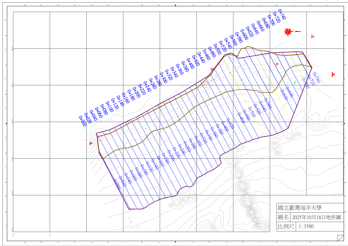
圖 4-1 2025 年 10 月 18 日監測地形
