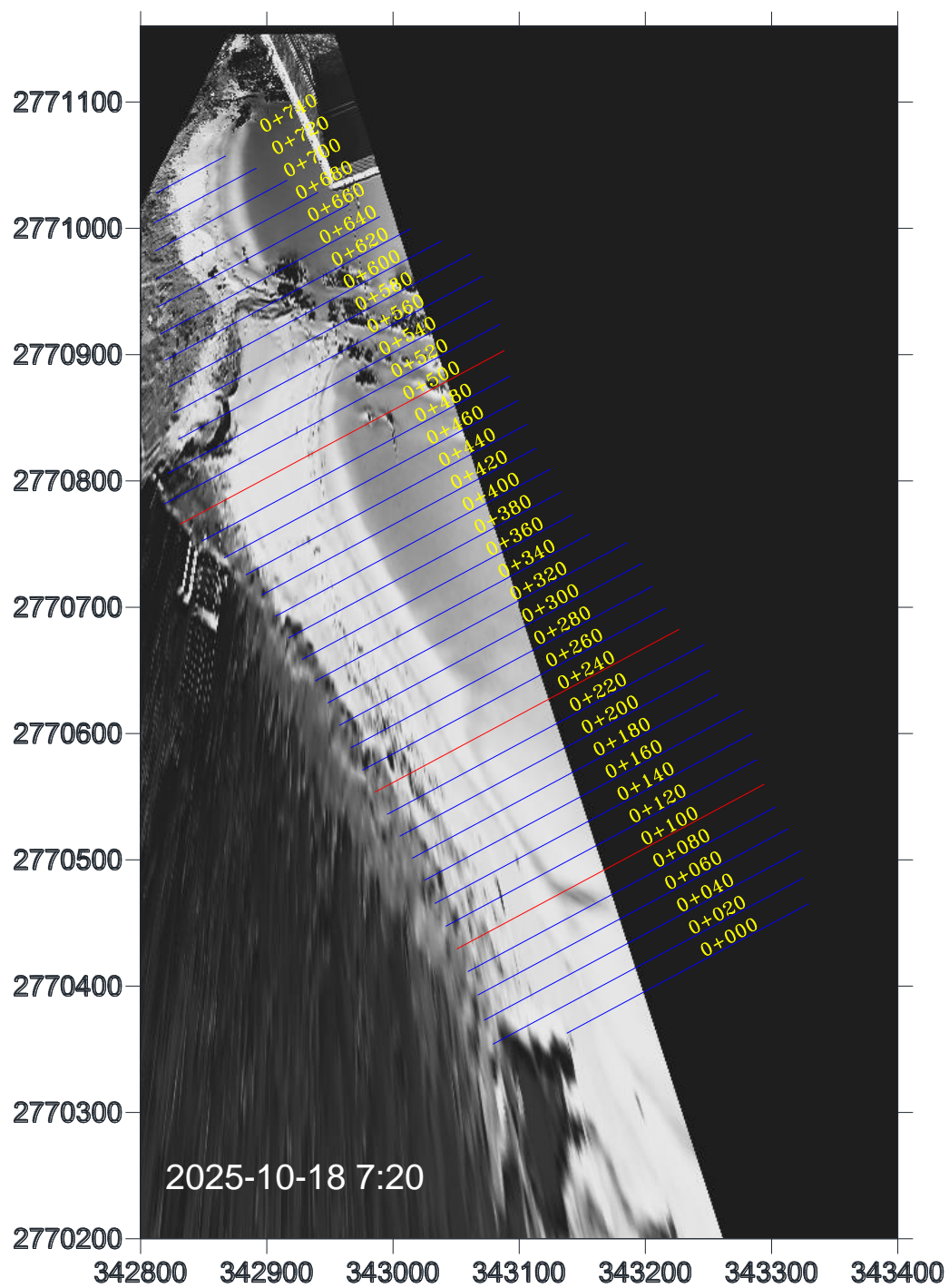
圖 4-19 鹽寮海岸地形影像全景圖(2025/10/18 7:20)
