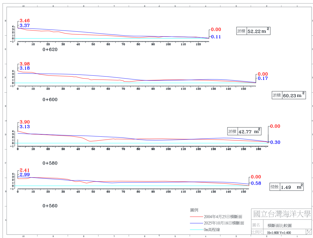
圖 4-4(c) 2025 年 10 月 18 日 A 監測區橫斷面比較圖
