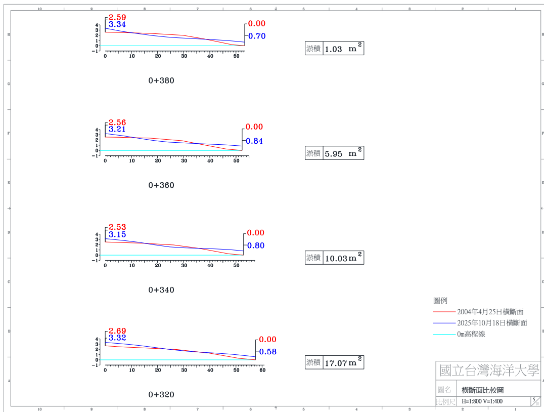
圖 4-4(f) 2025 年 10 月 18 日 A 監測區橫斷面比較圖
