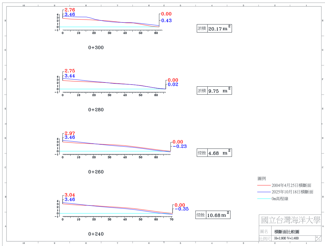
圖 4-4(g) 2025 年 10 月 18 日 A 監測區橫斷面比較圖
