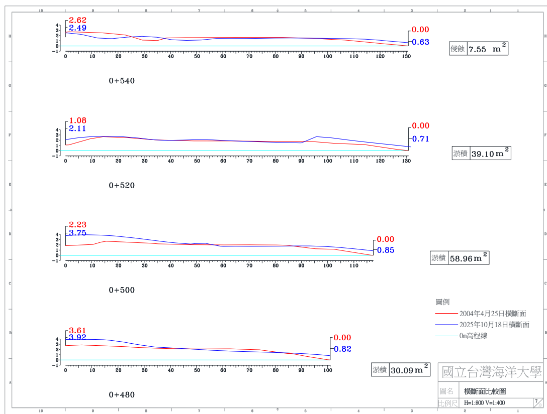
圖 4-4(d) 2025 年 10 月 18 日 A 監測區橫斷面比較圖
