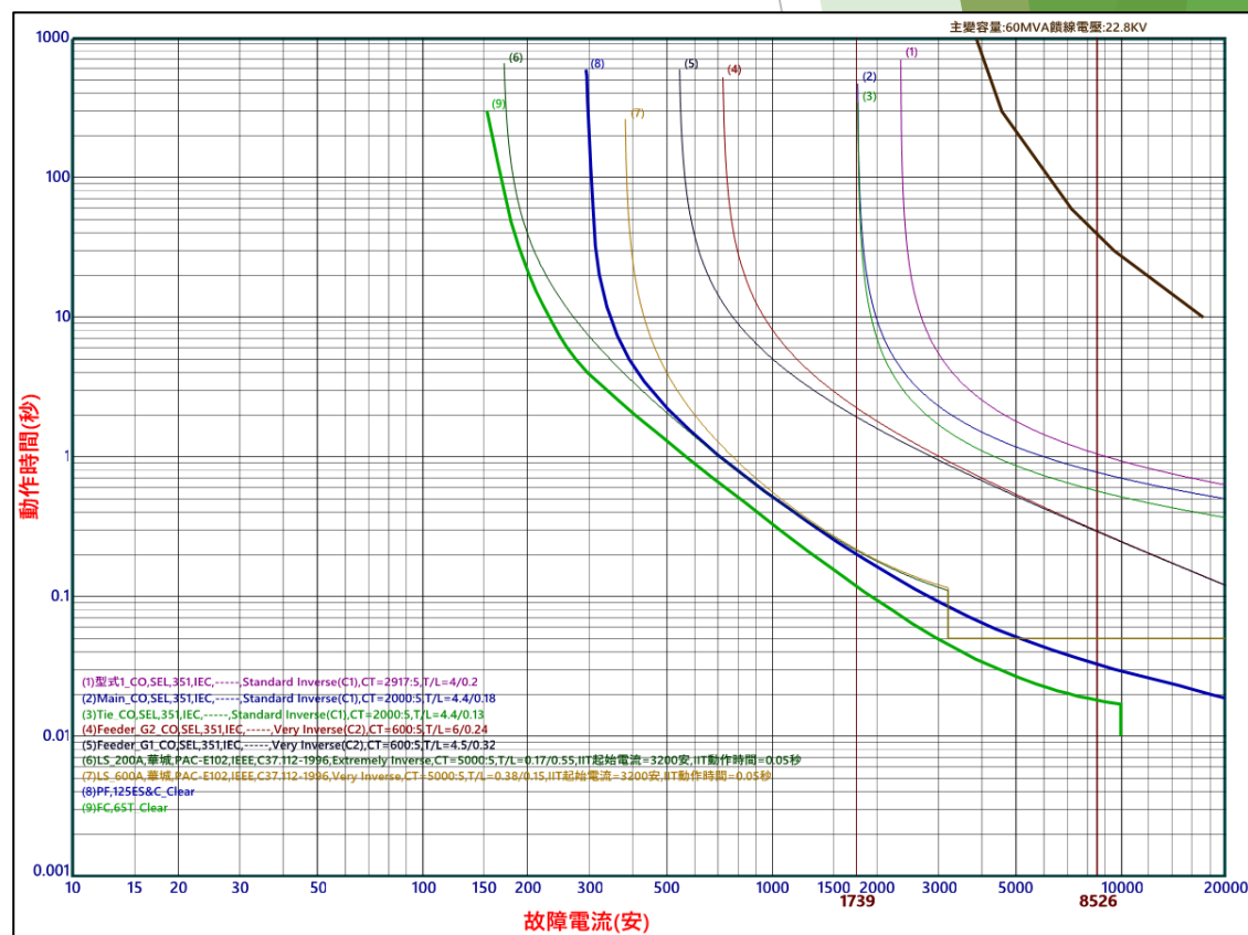
保護協調曲線圖
