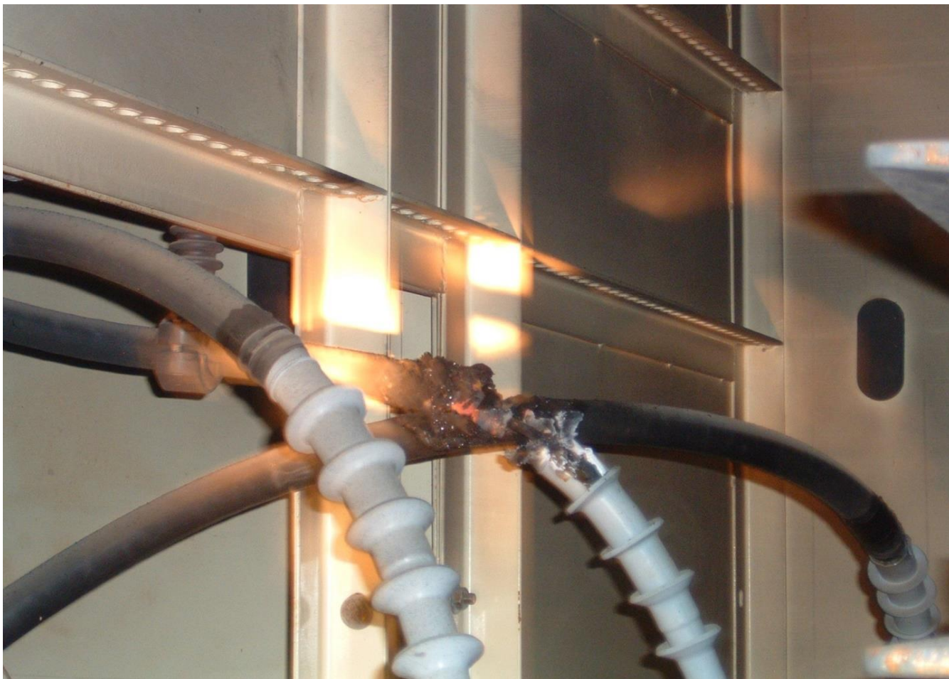
電纜終端接頭 外皮切開處即視同裸線
