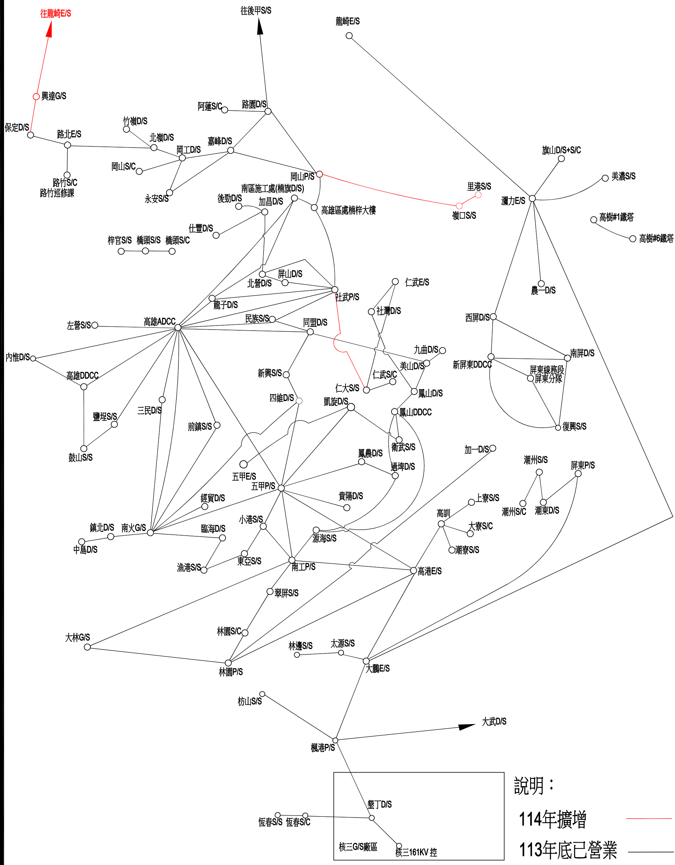
台電出租光纖網路系統圖_高雄市、屏東縣
