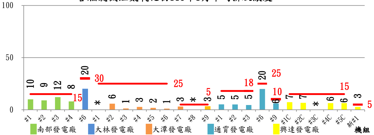
ppm(百萬分之一) 各燃氣機組氮氧化物115年1月平均排放濃度
