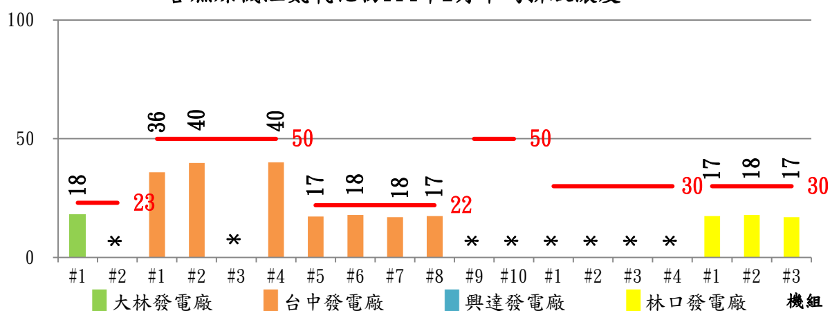
mg/m 3 (毫克/立方公尺) 各燃煤機組粒狀污染物114年2月平均排放濃度
