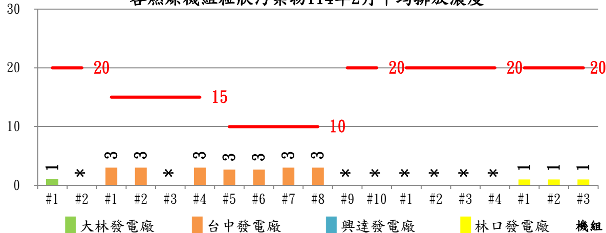
mg/m 3 (毫克/立方公尺) 各燃煤機組粒狀污染物114年2月平均排放濃度
