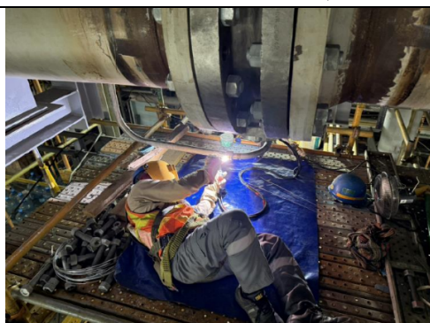
主發電設備工程 Unit 3 STB 配管
