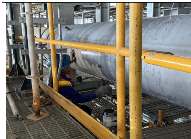
主發電設備工程 Unit 3 HRSG 配管
