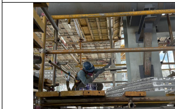
主發電設備工程 Unit 3 MPR 配管
