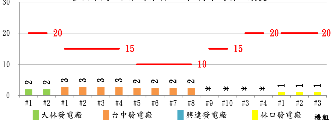
各燃煤機組粒狀污染物114年7月平均排放濃度
