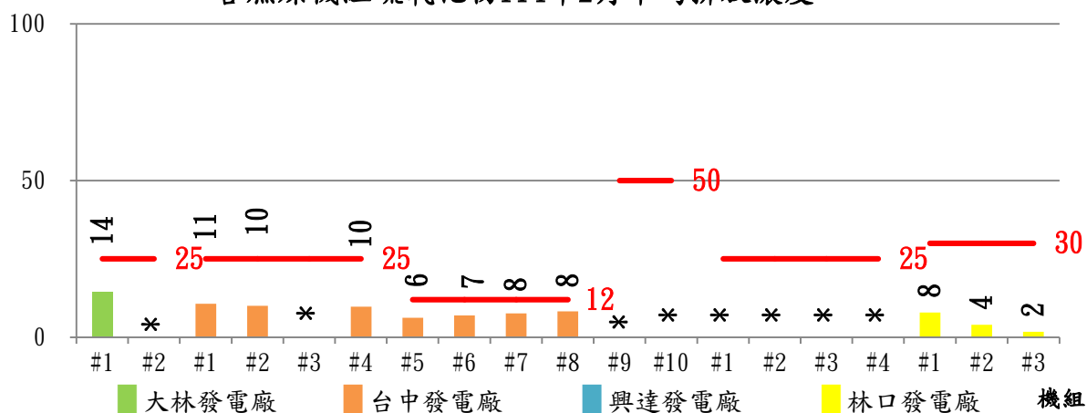
ppm(百萬分之一) 各燃煤機組氮氧化物114年2月平均排放濃度
