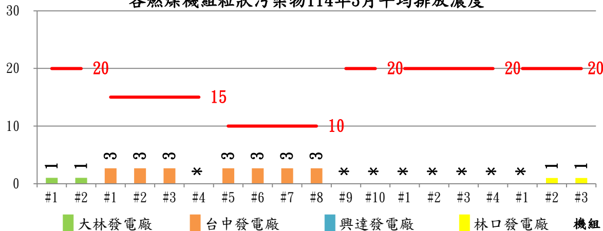
各燃煤機組粒狀污染物114年3月平均排放濃度
