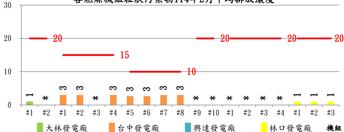
mg/m³(毫克/立方公尺) 各燃煤機組粒狀污染物114年2月平均排放濃度
