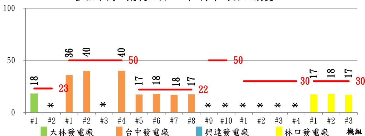
mg/m³(毫克/立方公尺) 各燃煤機組粒狀污染物114年2月平均排放濃度
