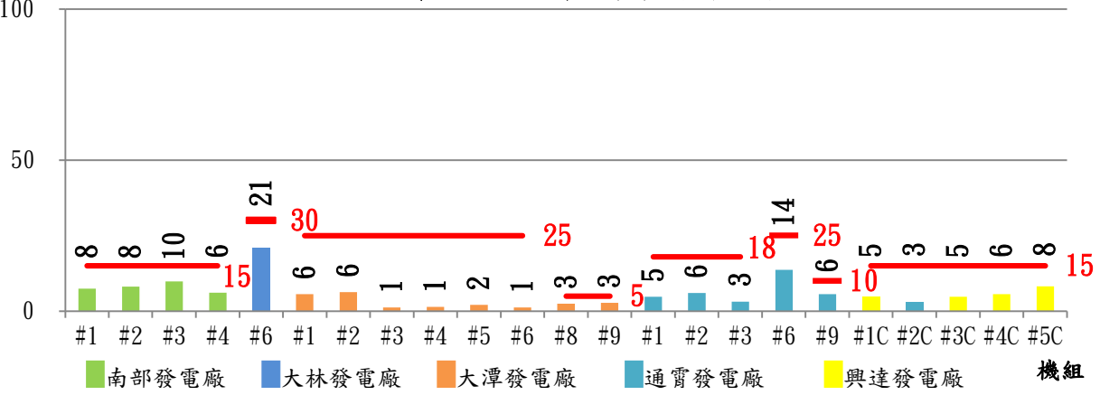
ppm(百萬分之一) 各燃氣機組氮氧化物114年6月平均排放濃度
