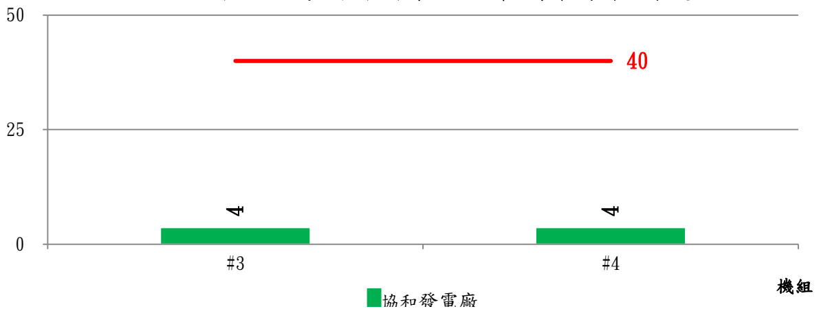
mg/m 3 (毫克/立方公尺) 各燃油機組粒狀污染物114年2月平均排放濃度
