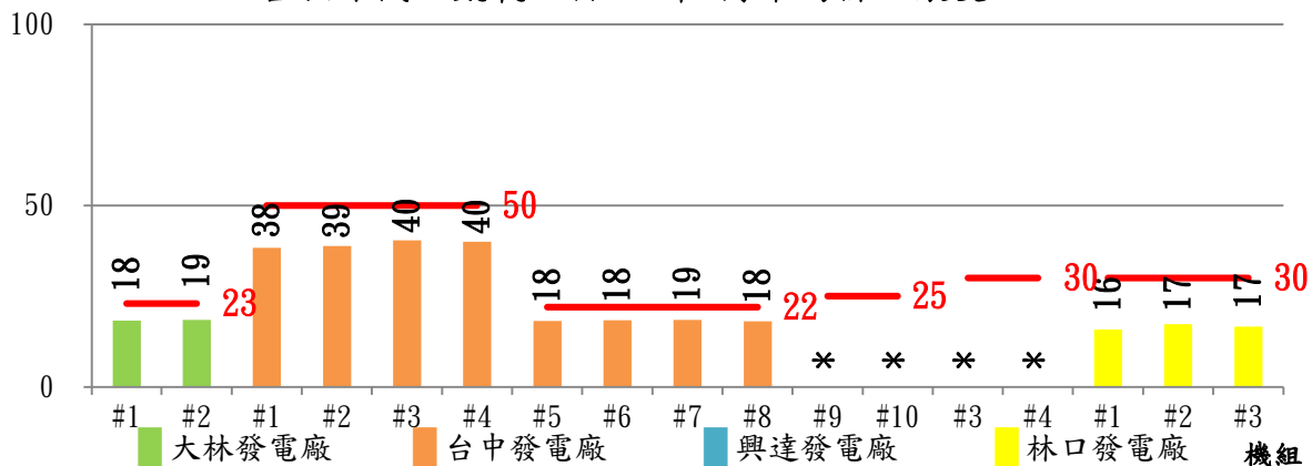
各燃煤機組粒狀污染物114年7月平均排放濃度
