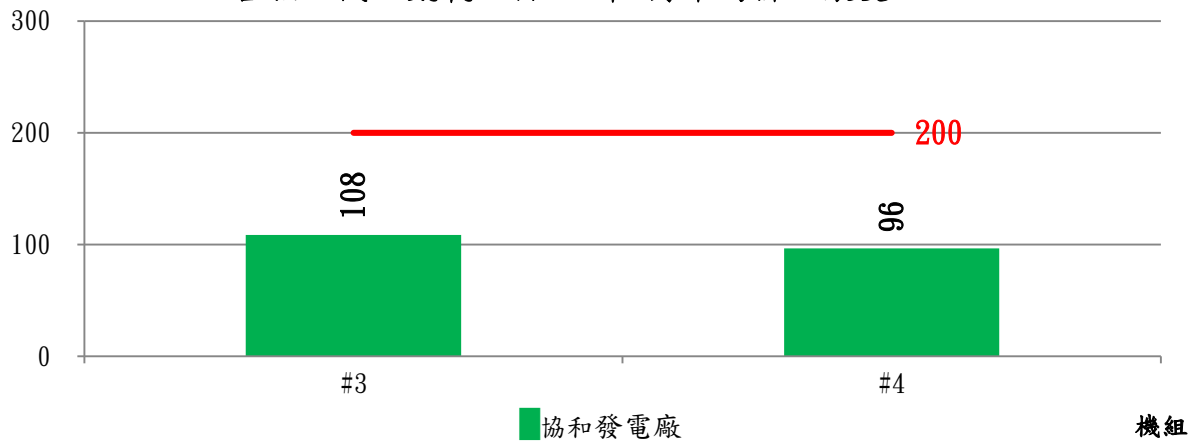
ppm(百萬分之一) 各燃油機組氮氧化物114年2月平均排放濃度
