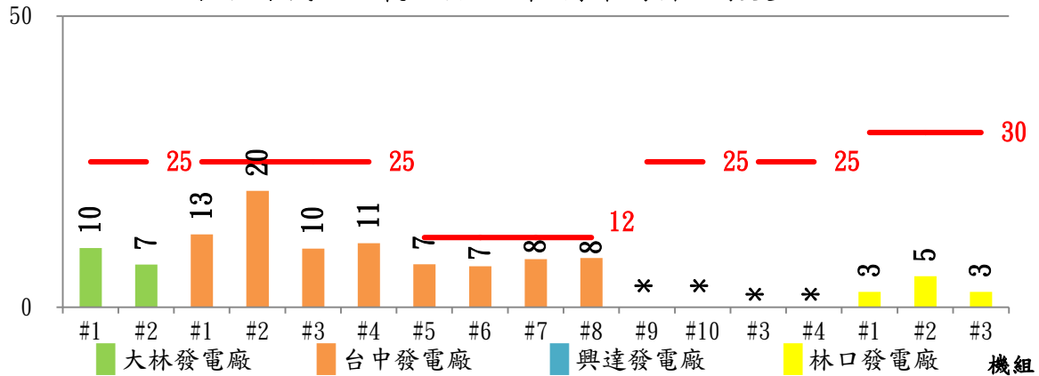
各燃煤機組氮氧化物114年7月平均排放濃度
