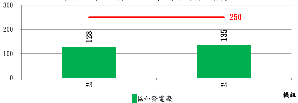
各燃油機組硫氧化物115年1月平均排放濃度
