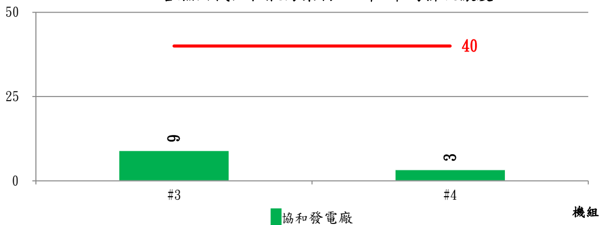
各燃油機組粒狀污染物115年1月平均排放濃度
