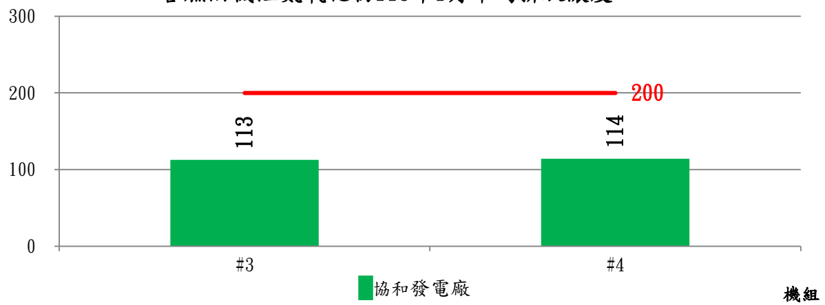
各燃油機組氮氧化物115年1月平均排放濃度
