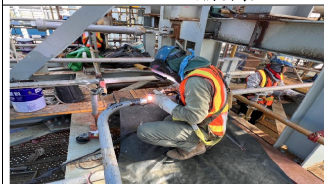
主發電設備工程 Unit 3 MPR 配管
