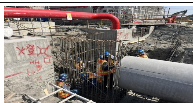
主發電設備工程 排水系統施作
