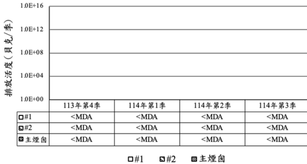
圖五 核一廠放射性廢氣排放統計圖 (氮-13)
