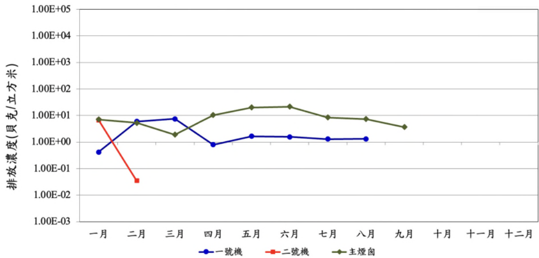
圖七 核一廠各廢氣排放源-總排放濃度統計圖
