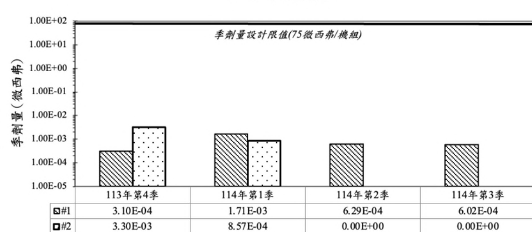
圖十四 核一廠放射性廢氣途徑關鍵群體 器官等價劑量
