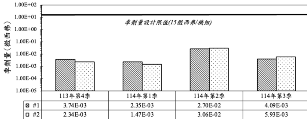
圖十五 核一廠放射性廢水途徑關鍵群體 有效劑量
