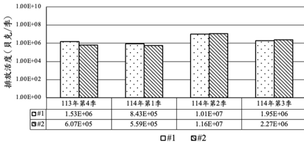
圖八 核一廠放射性廢水排放統計圖 (分裂及活化核種)
