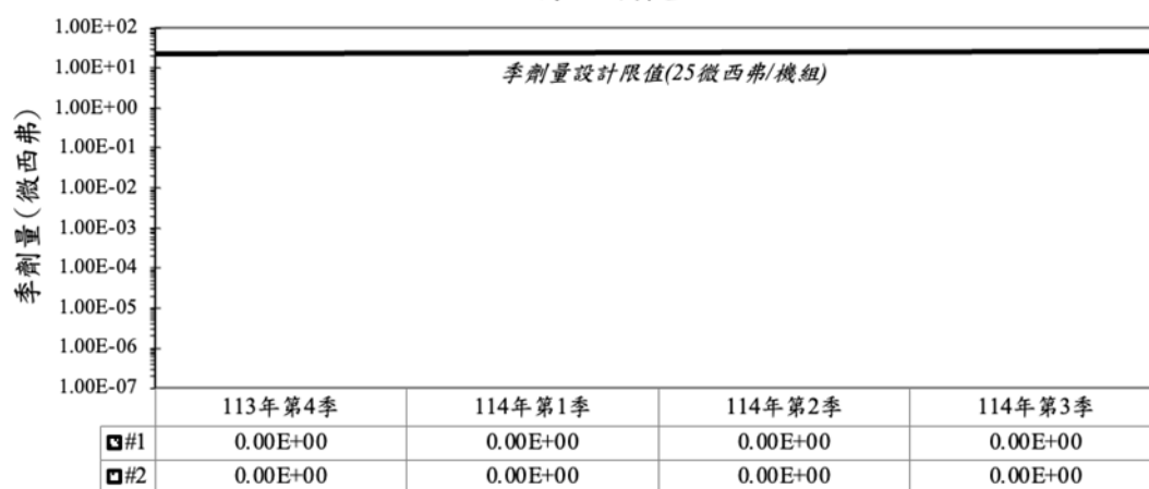
圖十三 核一廠放射性廢氣途徑關鍵群體 有效劑量
