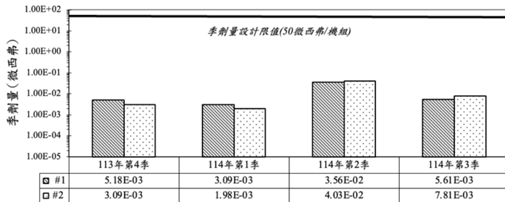
圖十六 核一廠放射性廢水途徑關鍵群體 器官等價劑量
